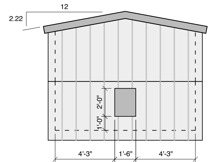
Right Elevation
